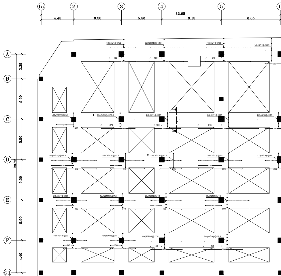
پلان آرماتور برشی فنداسیون (جهت طولی) SC:1/100
