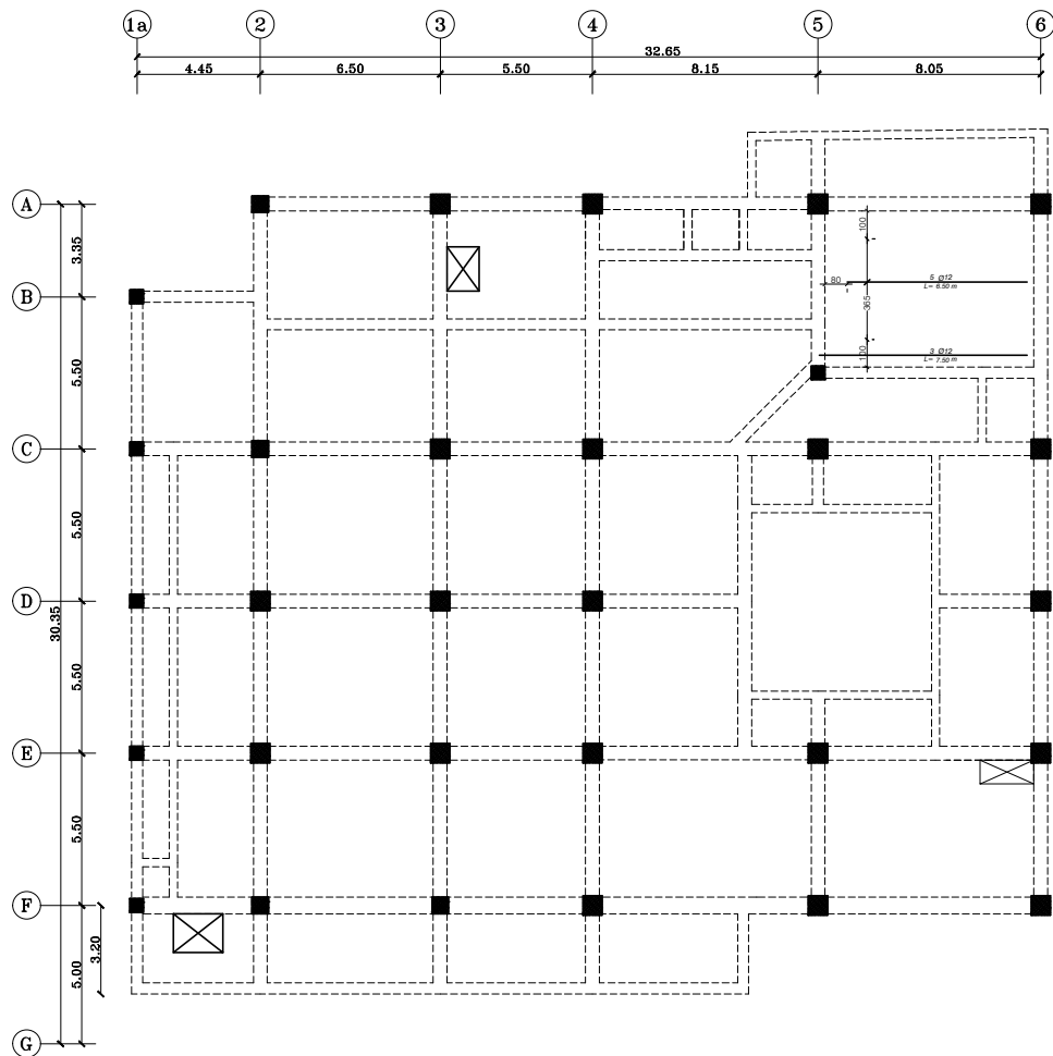
پلان آرماتورگذاری تقویتی ملولی (تحتانی) پلان آرماتورگذاری ملالی در تراز +۰.۳۸۸
