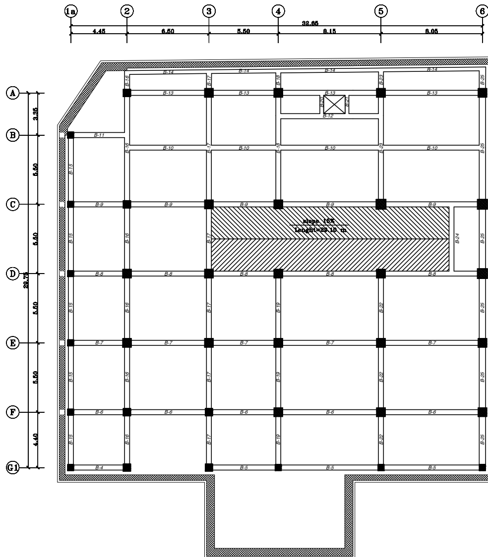
پلان تیرریزی تراز ۲/۲۵
