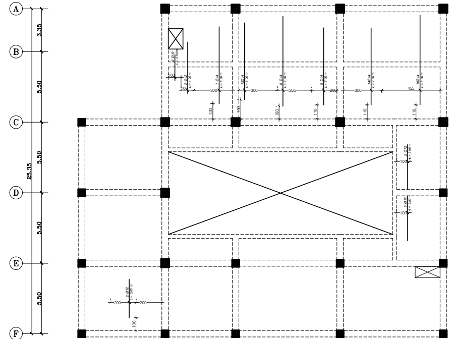
پلان آرماتورگذاری تقویتی عرضی (تحتانی) پلان آرماتورگذاری مال در تراز +۱۹۷۰
