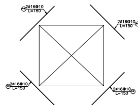
تقویت دال در محل بازشو
