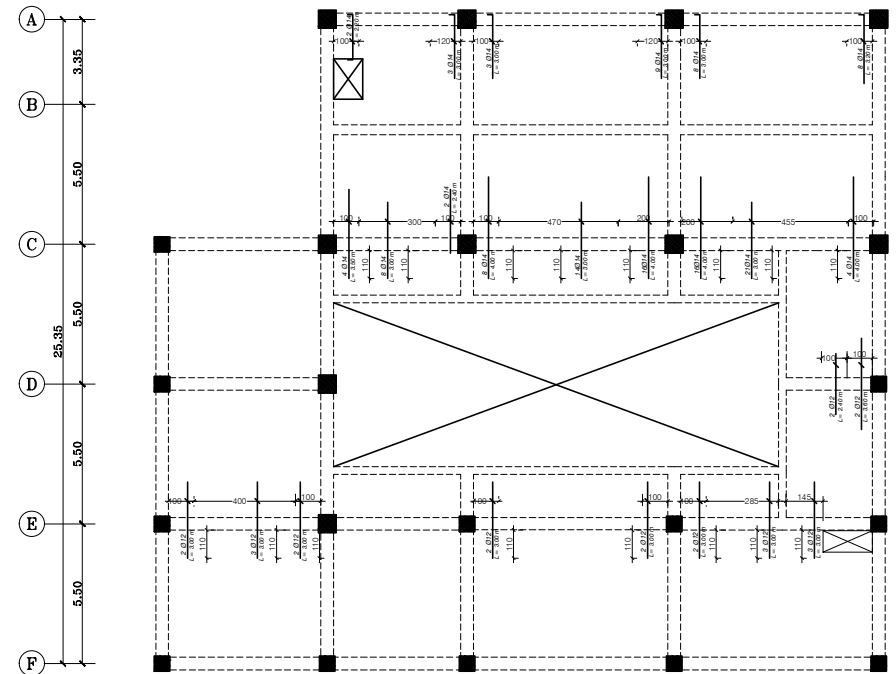
پلان آرماتورگذاری تقویتی طولی (فوقانی) پلان آرماتورگذاری دال در تراز +۱۷۷۰
