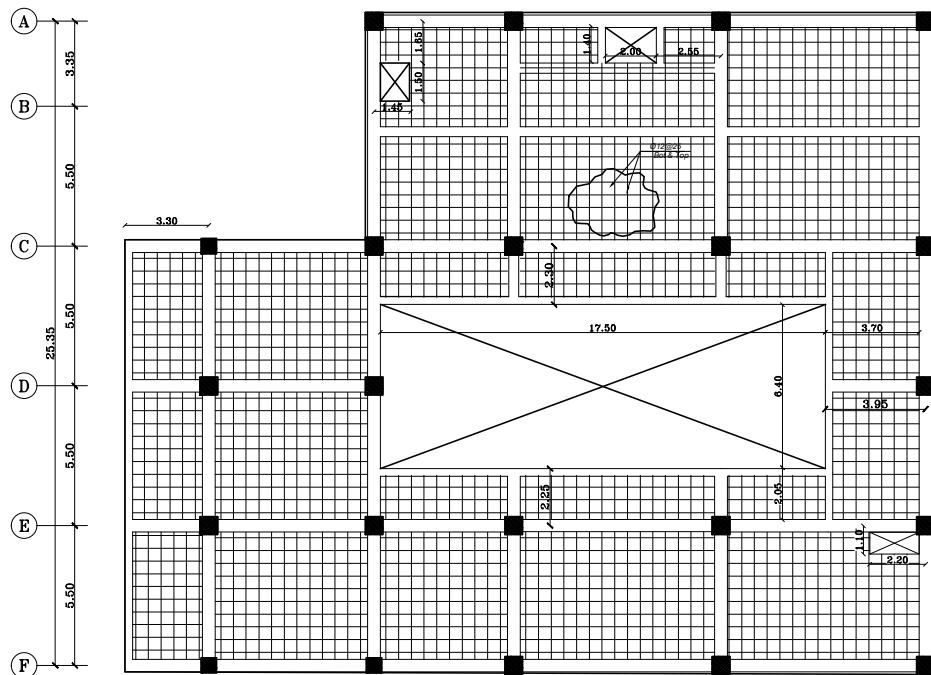
پلان آرماتورگذاری دال در تراز +V/82
