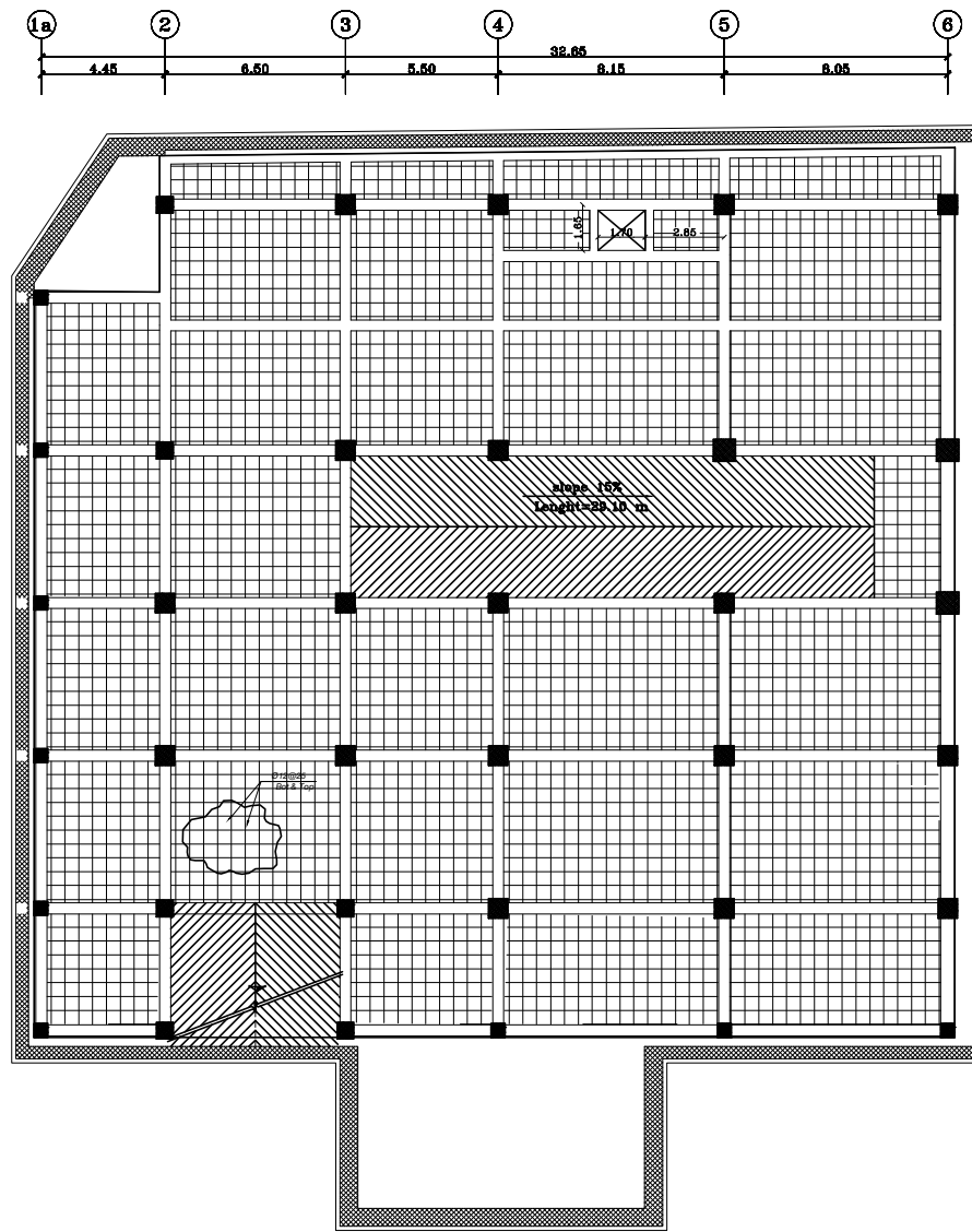
پلان آرماتورگذاری دال در تراز ۳/۴۵
