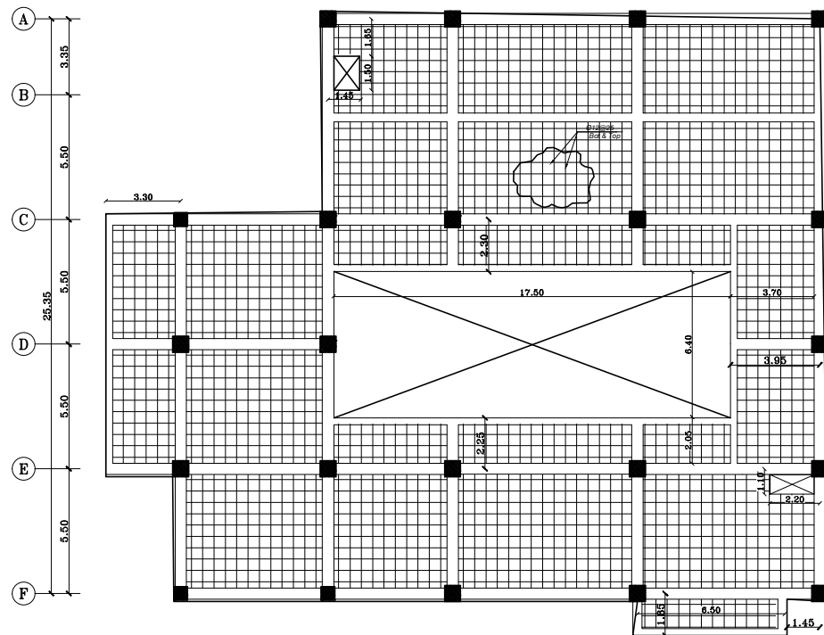
پلان آرماتورگذاری دال در تراز +V/84
