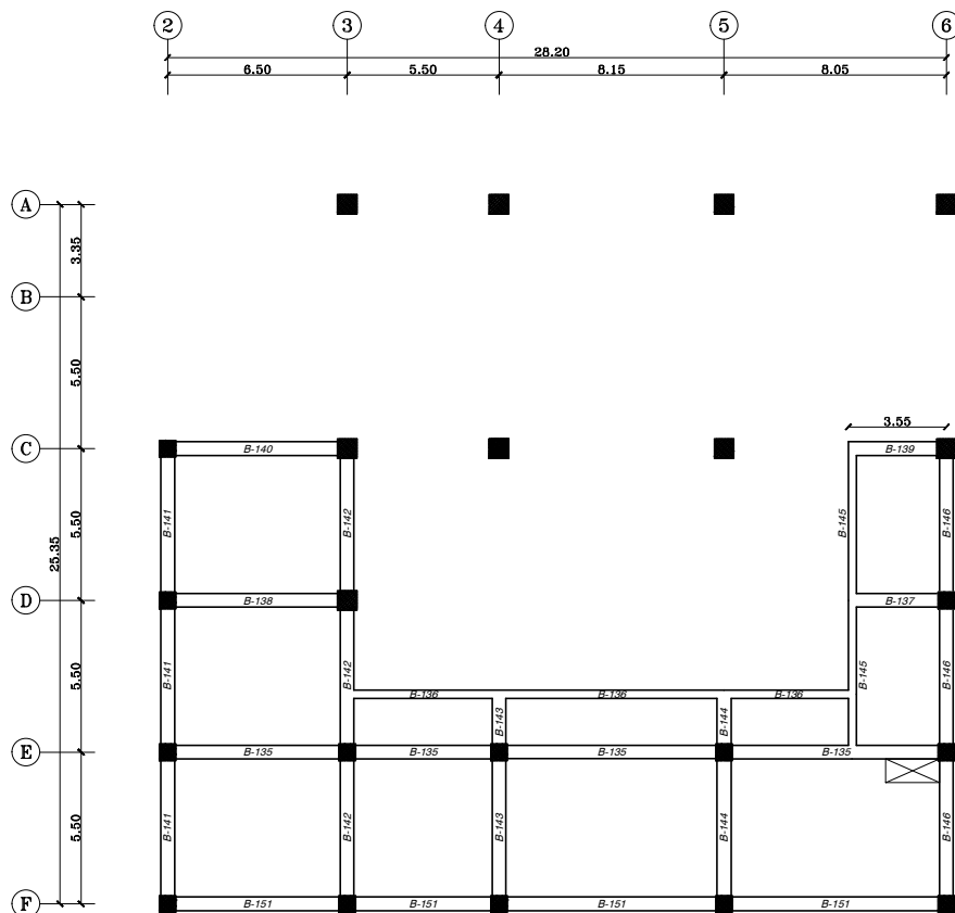
پلان تیریزی تراز ۲۴/۱۶
