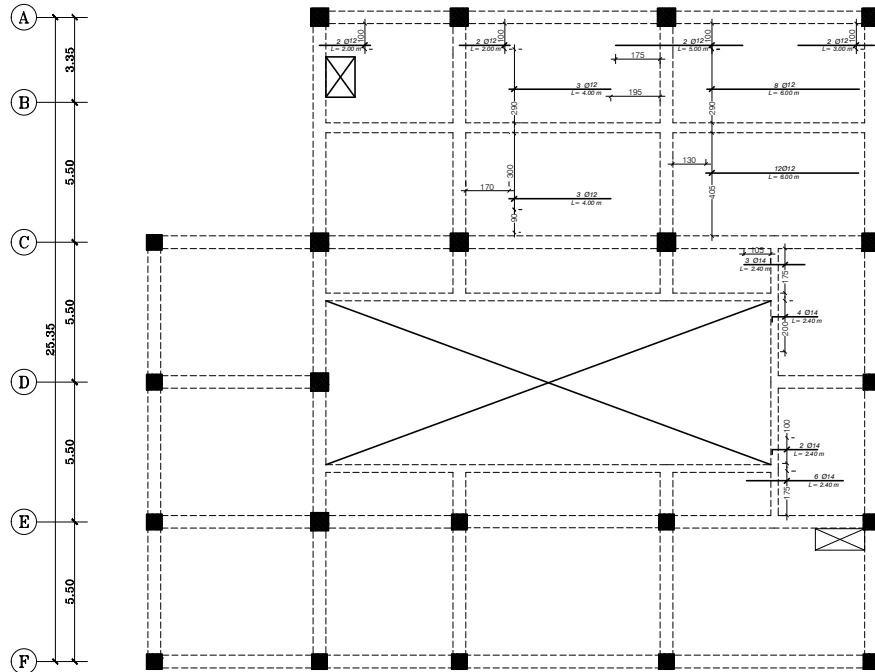
پلان آرماتورگذاری تقویتی طولی (تحتانی) پلان آرماتورگذاری مال در تراز +۱۹۷۰
