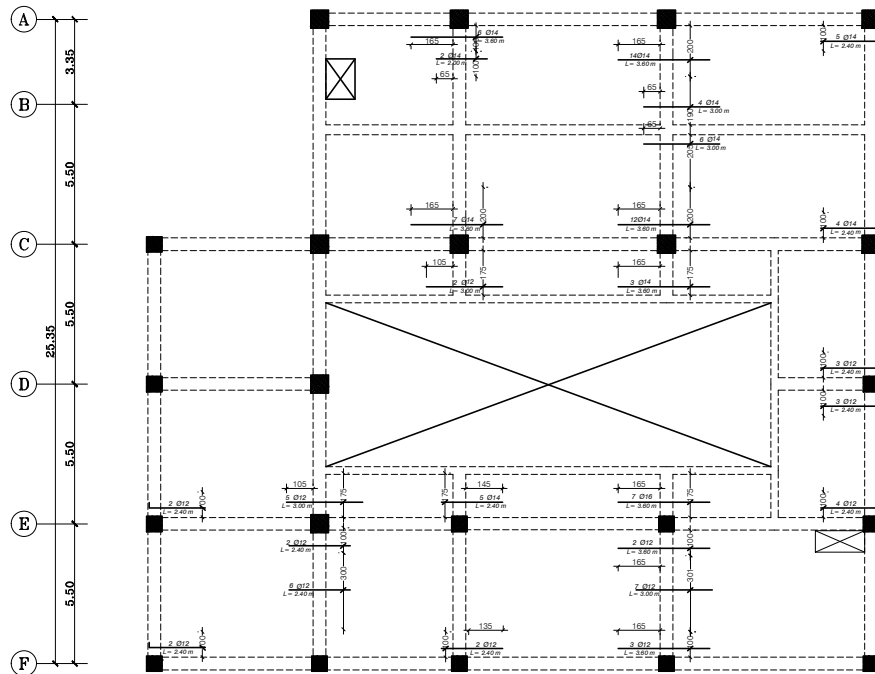
پلان آرماتورگذاری تقویتی عرضی (فوقانی) پلان آرماتورگذاری دال در تراز +۱۷۷۰
