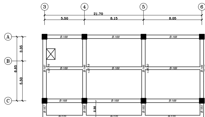
پلان تیریزی سقف آمفی تئاتر
