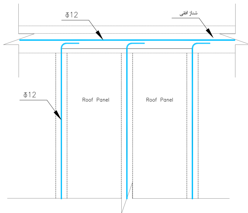
جزئیات اجرای مهار میلگرد شناژ بین پنل های سقف در شناژ افقی
