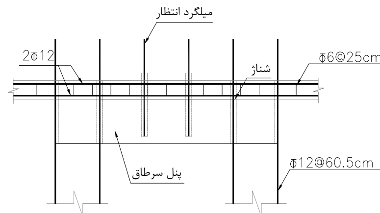
جزئیات اجرای ادامه دیوار در طبقه فوقانی
