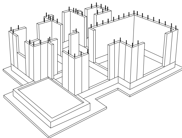
پلان اتصال پانل های دیواری
