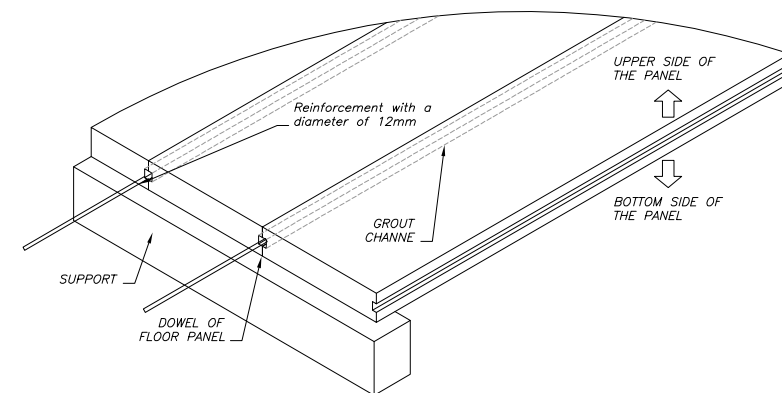
اتصال پانل سقف
