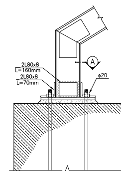
جزئیات اتصال شمشیری پله به فنداسیون
