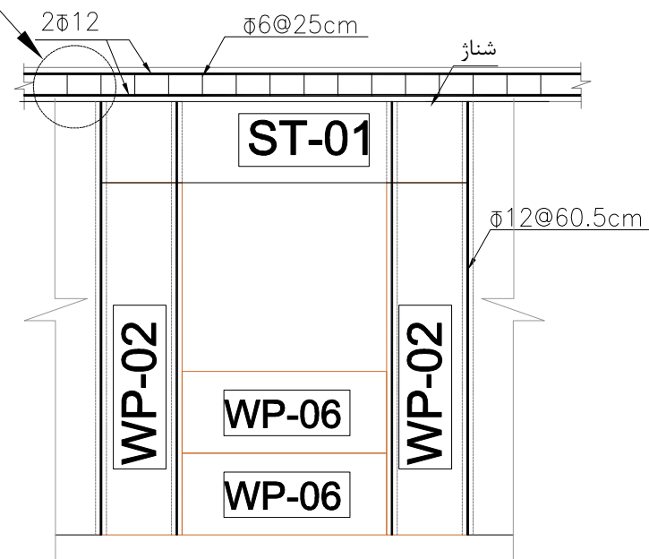
جزئیات اجرای سرطاق
