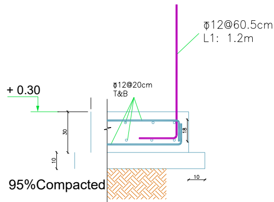
Sec A-A SC: 1:20
